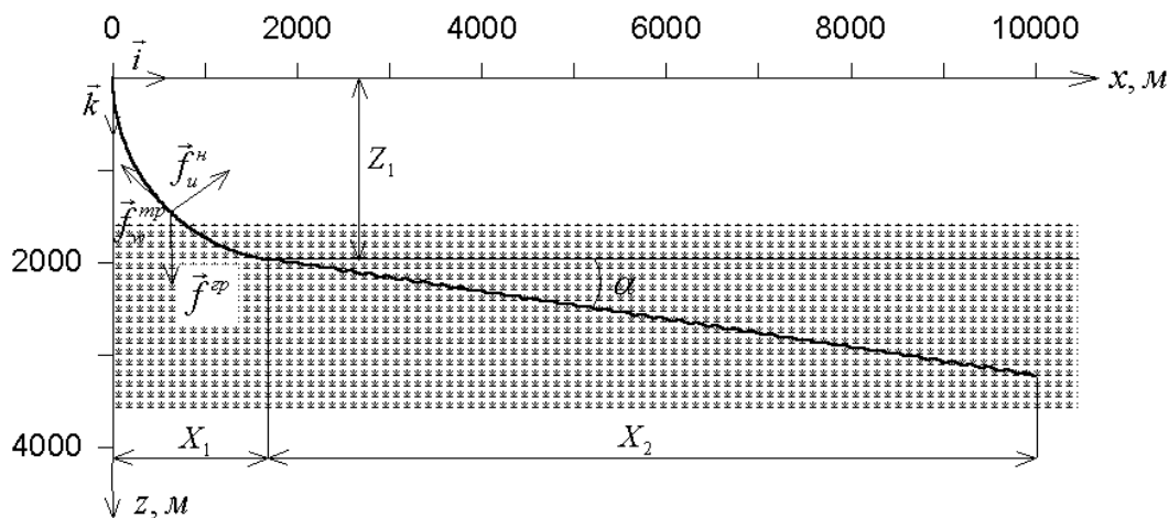
Рисунок 1 — Геометрична схема похило-скерованої свердловини
