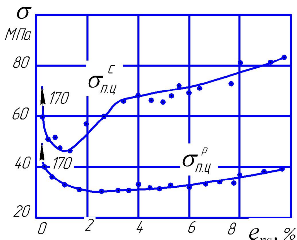
Рисунок 15 — Залежності \sigma_{nc}^c і \sigma_{nc}^p сталі 17Г1С від величини наклепу стиском e_{nc}
