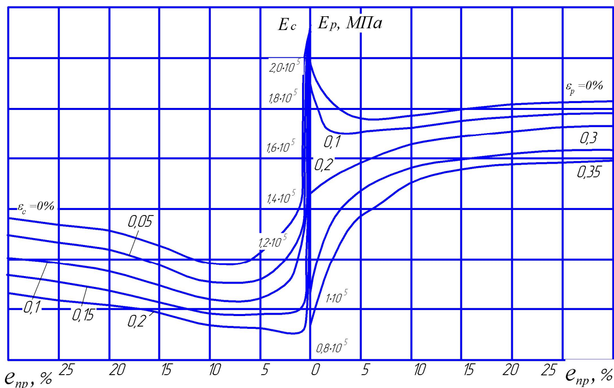
Рисунок 6 — Залежності січних модулів розтягу E_p і стиску E_c сталі 17Г1С від величини попередньої пластичної деформації розтягом e_{np} за різних значень відносного видовження \epsilon_p і відносного стиску \epsilon_c ( \sigma_c = -200 \text{ МПа} )
