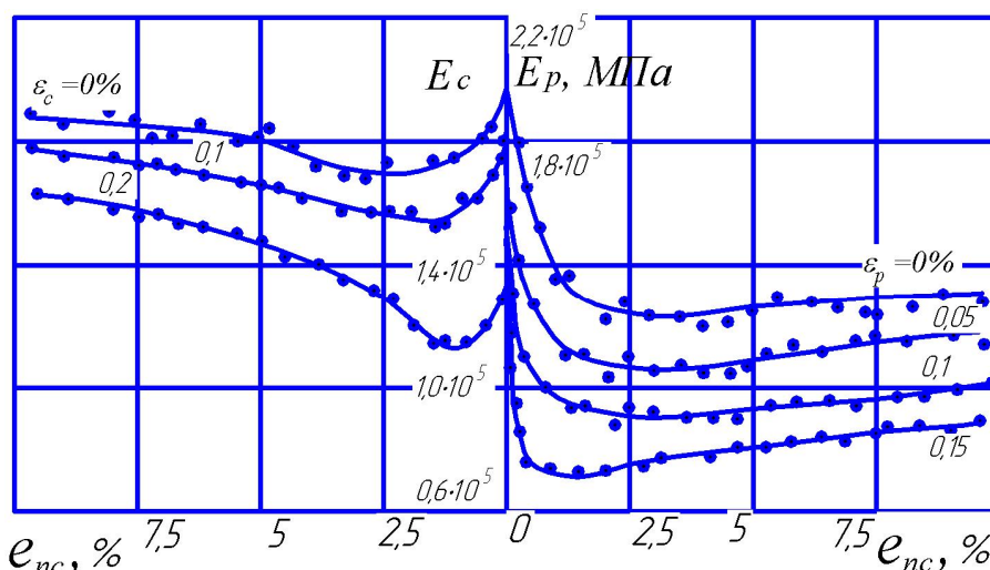
Рисунок 14 — Залежність січних модулів розтягу E_p і стиску E_c сталі 17Г1С від величини попередньої пластичної деформації стиском e_{nc} за різних значень відносного видовження \epsilon_p і відносного стиску \epsilon_c
