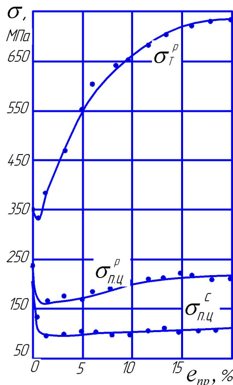
Рисунок 12 — Залежності \sigma_{nc}^p , \sigma_{nc}^c і \sigma_T^p сталі 17Г1С від величини наклепу розтягом
