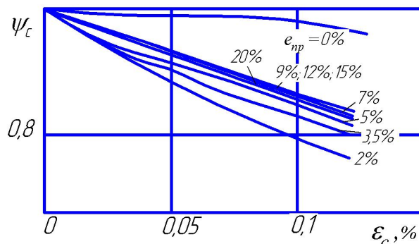
Рисунок 5 — Залежність відносної зміни модуля стиску E_c сталі 17Г1С від величини відносного стиску \varepsilon_c за різних значень попередньої пластичної деформації e_{np} ( \sigma_c = -100\text{МПа} )
