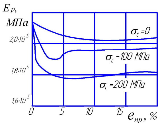
Рисунок 7 — Вплив попереднього пластичного деформування e_{np} і величини напружень стиску на характер кривих E_p (за \epsilon_p = 0 )
