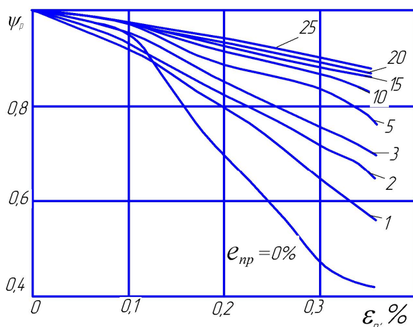
Рисунок 10 — Вплив проміжного стиску ( \sigma_c = -200 \text{ МПа} ) на залежність відносної зміни модуля E_p сталі 17Г1С від величини відносного видовження \varepsilon_p за різних значень попередньої пластичної деформації e_{np}
