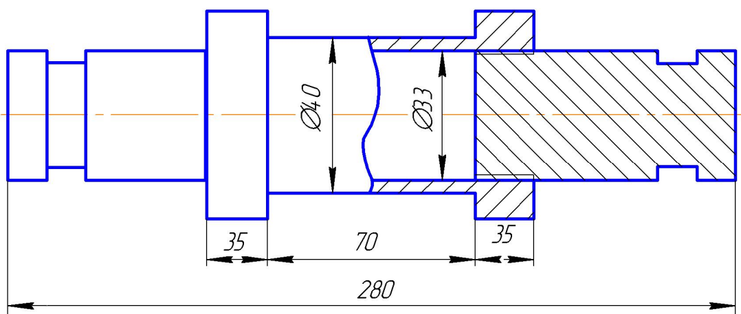
Рисунок 13 — Схематичне зображення зразка для механічних випробовувань на «стискання-розтягування»
