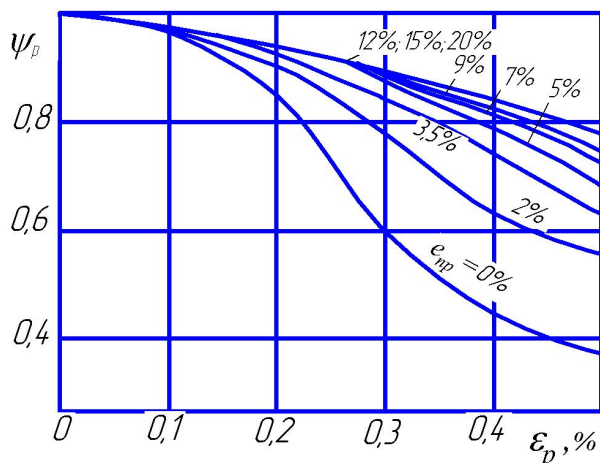
Рисунок 4 — Вплив проміжного стиску ( \sigma_c = -100\text{МПа} ) на залежність відносної зміни модуля E_p сталі 17Г1С від величини відносного видовження \varepsilon_p за різних значень попередньої пластичної деформації e_{np}
