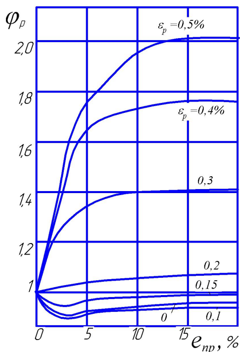
Рисунок 2 — Вплив проміжного стиску ( \sigma_c = -100\text{МПа} ) на залежність відносної зміни модуля E_p сталі 17Г1С від величини попередньої пластичної деформації e_{np} за різних значень відносного видовження \varepsilon_p
