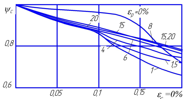
Рисунок 11 — Залежність відносної зміни модуля стиску E_c сталі 17Г1С від величини відносного стиску \varepsilon_c за різних значень попередньої пластичної деформації e_{np} ( \sigma_c = -200 \text{ МПа} )
