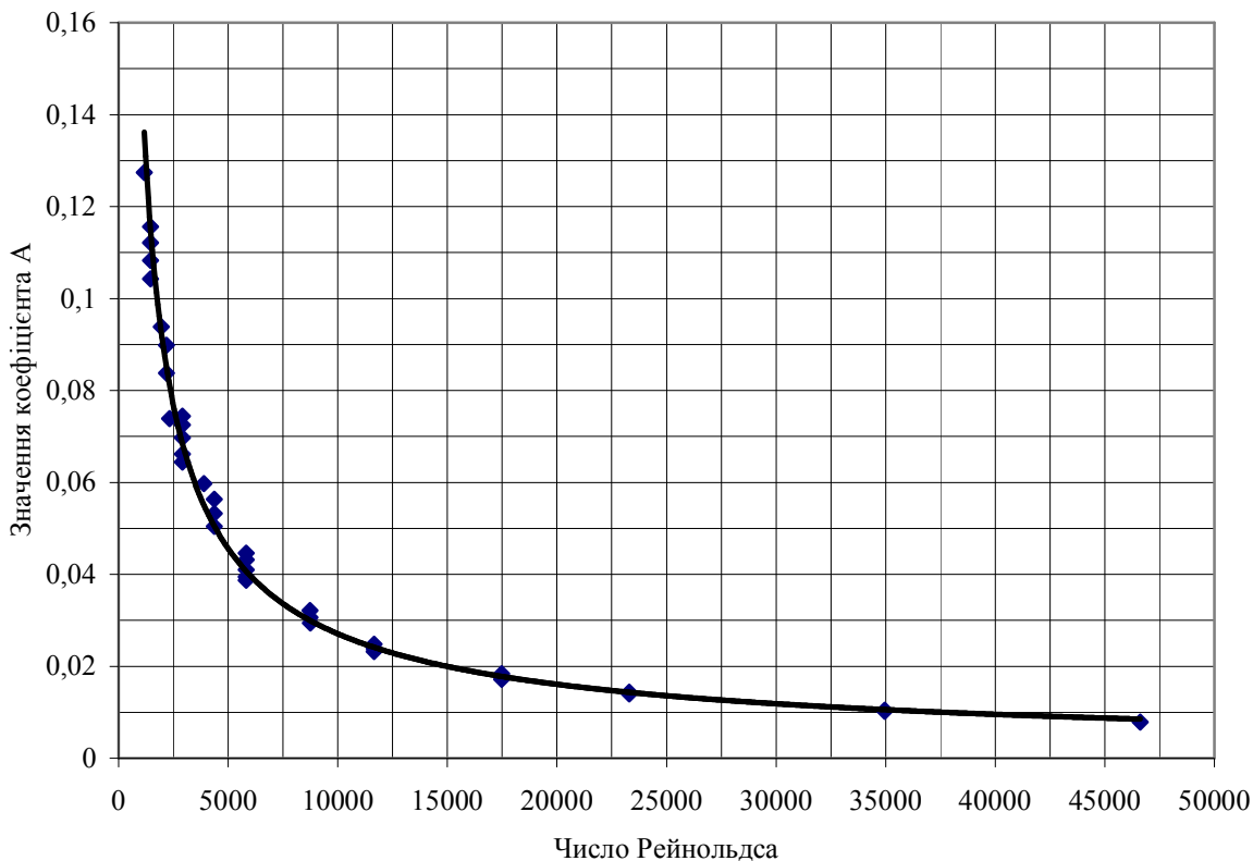
Рисунок 5 — Залежність коефіцієнта А від числа Рейнольдса у математичній моделі для коригувального коефіцієнта збільшення гідравлічного опору у разі перекачування нелінійно-в'язкопластичної рідини у турбулентному режимі
