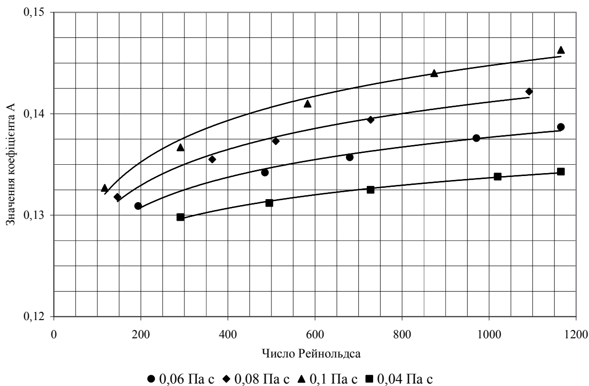
Рисунок 7 — Залежність коефіцієнта А від числа Рейнольдса і коефіцієнта консистентності у математичній моделі для коригувального коефіцієнта збільшення гідравлічного опору у разі перекачування нелінійно-в'язкопластичної рідини у ламінарному режимі
