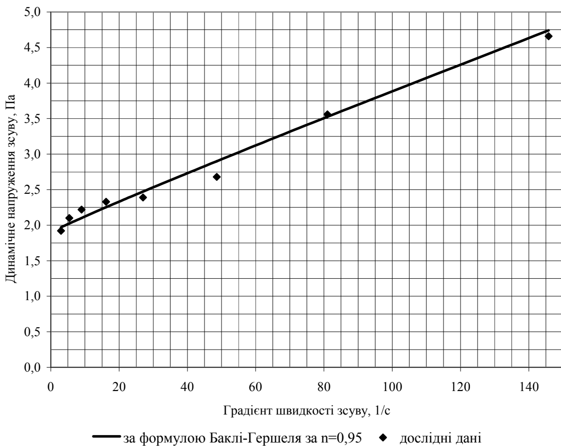
Рисунок 2 — Залежнiсть динамiчного напруження зсуву вiд градiєнта швидкостi зсуву для долинської нафти, що перекачувалась у листопадi 2008 р. (температура пiдiгрiву 60°C, робоча температура нафти 25°C)
