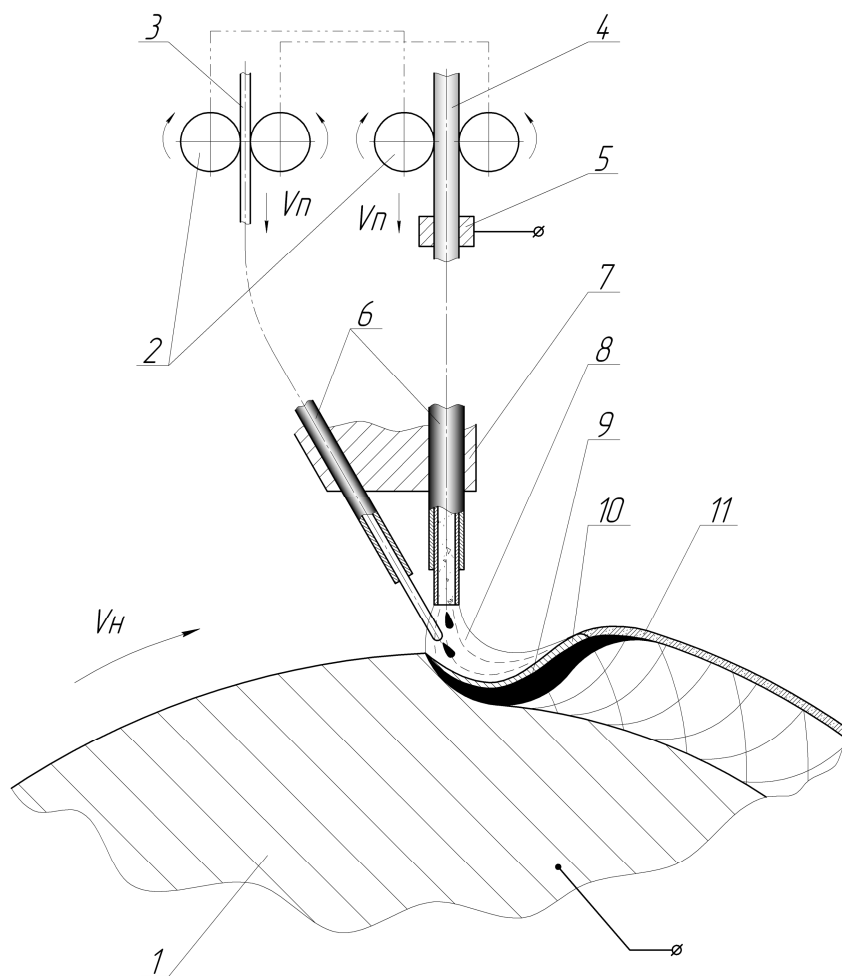
1 – опорний каток (наплавлювана деталь); 2 – подаючі ролики; 3 – присадковий матеріал (електродний дріт); 4 – самозахисний порошковий дріт; 5 – струмопровід; 6 – направляючі дротів (мундштуки); 7 – кронштейн; 8 – дуга; 9 – наплавлювальна ванна; 10 – розплавлений шлак; 11 – шлакова кірка; V_n – швидкість наплавлення (обертання деталі); V_p – швидкість подавання електродів
