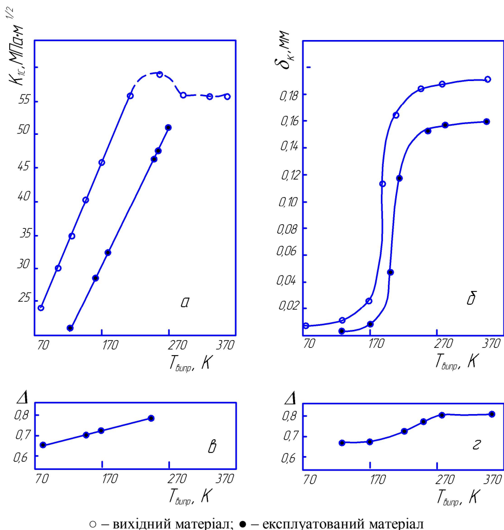
Рисунок 1 – Зміна характеристик в'язкості руйнування K_{1C} (а) та \delta_K (б) сталі 17Г1С залежно від температури випробувань та показник відносних змін \Delta характеристик K_{1C} (в) і \delta_K (г) експлуатованої сталі, віднесених до їх початкового значення
