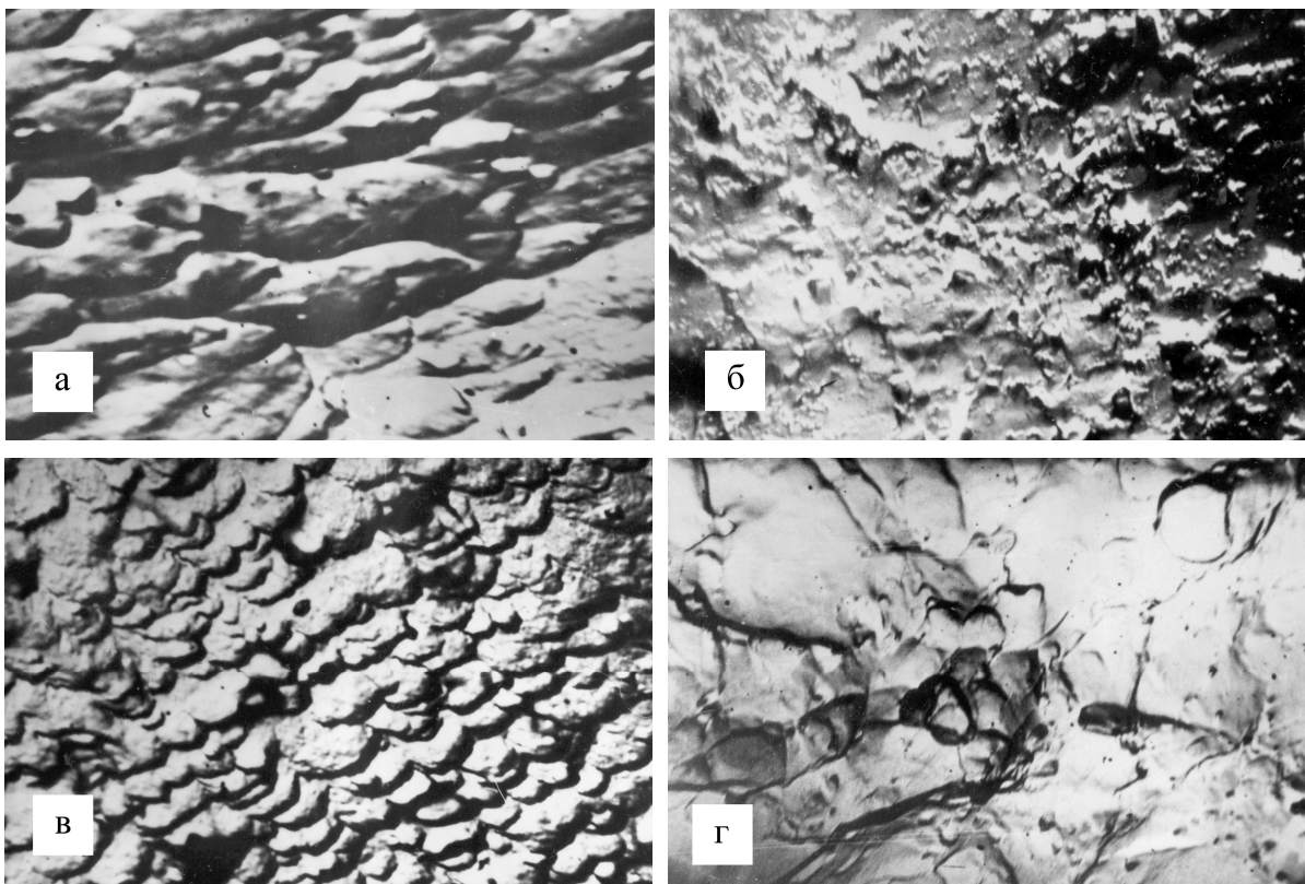
а,б – зразки, вирізані з контрольних труб; в,г – зразки, вирізані з експлуатованих труб; а,в – випробовування на повітрі; б,г – випробовування у дистильованій воді ( T_{випр}=293K . Масштаб 1x2700)
