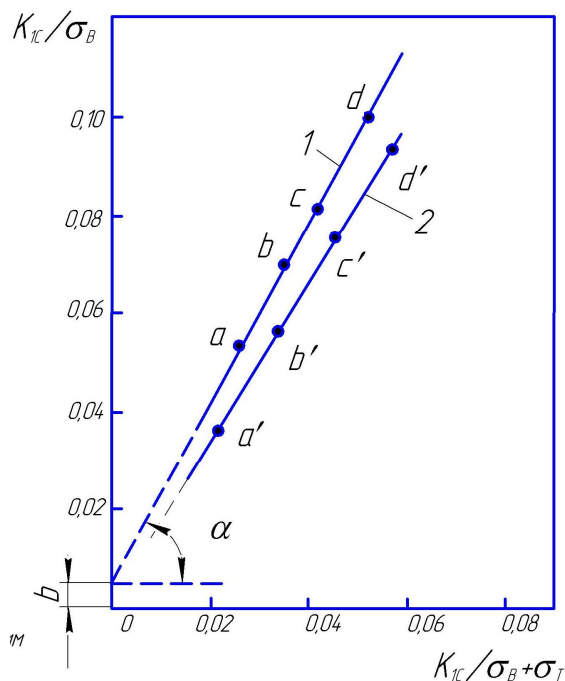
Рисунок 7 – Залежності K_{1C}/\sigma_B - K_{1C}/\sigma_B + \sigma_T за різних температур випробувань неексплуатованої (1) та експлуатованої (2) сталей 17Г1С
