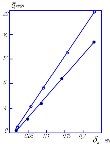
Рисунок 6 – Залежність ширини зони витяжки \bar{a} від \delta_{к\partial} при зміні температур випробувань для сталі 17Г1С для зразків, вирізаних з контрольних ( \circ ) і експлуатованих ( \bullet ) труб
