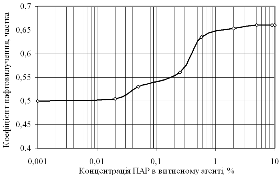
Рисунок 3 – Залежність коефіцієнта нафтовилучення від концентрації ПАВ у витісному агенті
