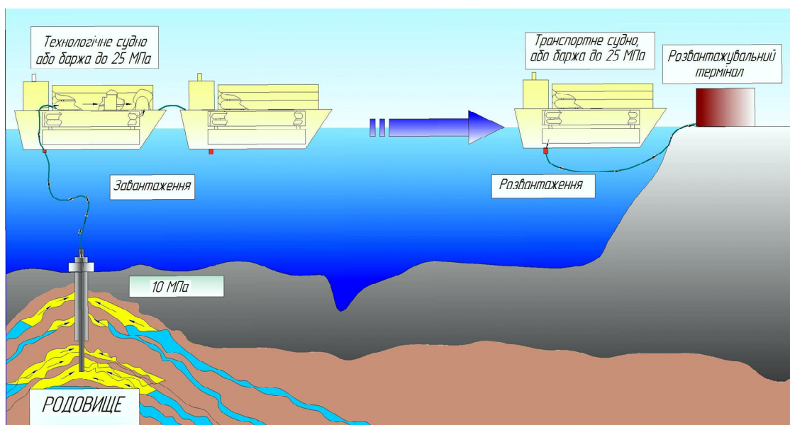
Рисунок 4 – Технологічний ланцюг технології CNG
