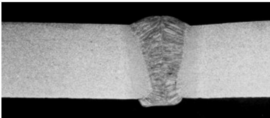
Рисунок 2 – Макрошліф зварного з'єднання товщиною 10 мм, виконаного за один прохід без попереднього розкриття кромки зварюванням в захисних газах дротом суцільного перерізу з активацією дуги [16]
