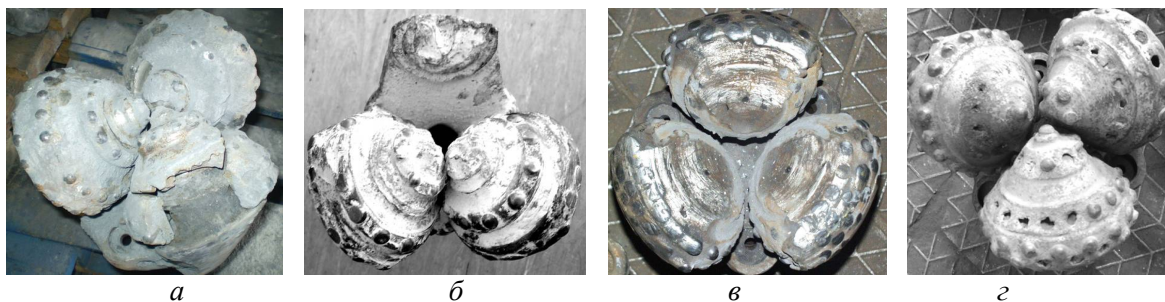
а – розколювання тіла шарошки, б – відламування цапфи лапи, в – заклинювання опор і зупинення обертання шарошок,
