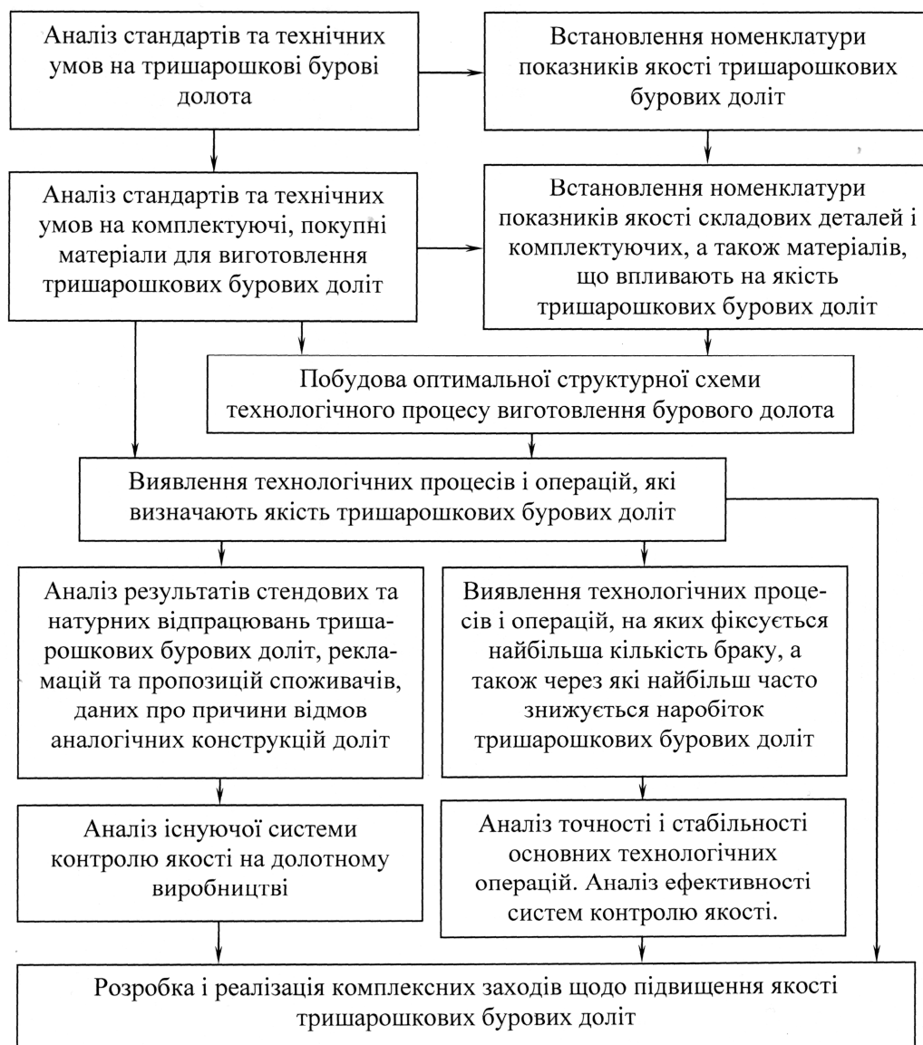
Рисунок 4 – Схема виявлення параметрів елементів технологічної системи, які визначають якісні показники тришарошкових бурових доліт
