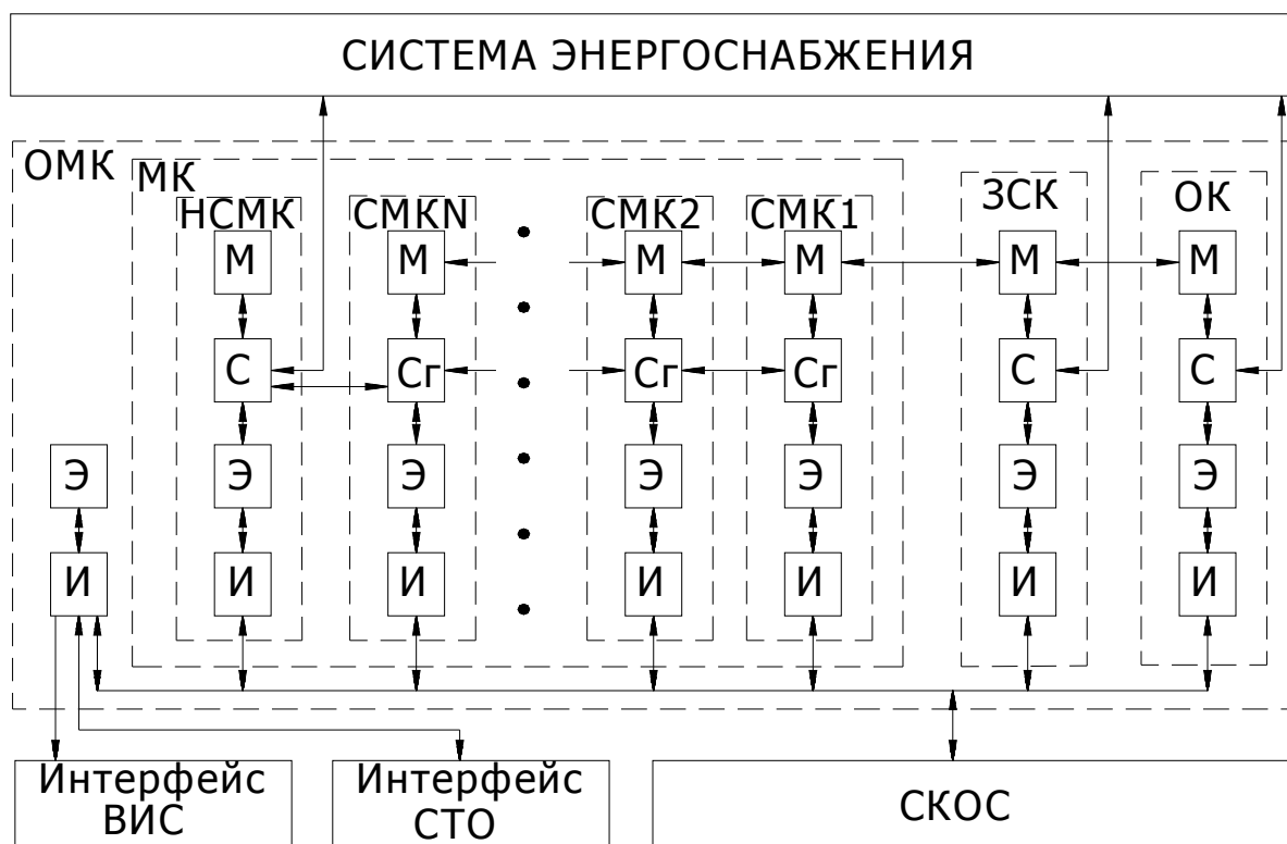
Рисунок 1 – Функционально-структурная схема ОмК как мехатронной системы
