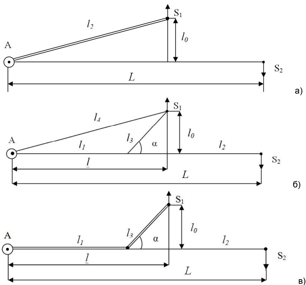
a – радіальна схема; б – схема двобічного живлення; в – схема магістрального живлення з реконструкцією головної ділянки
