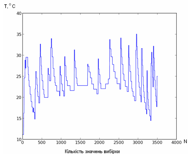
Рисунок 4 – Графік температури працюючих колодок упорного підшипника нагнітача ГПА, що аналізувалась
