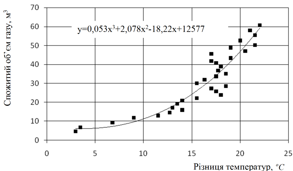
Рисунок 1 – Вплив температурних режимів на споживання газу
