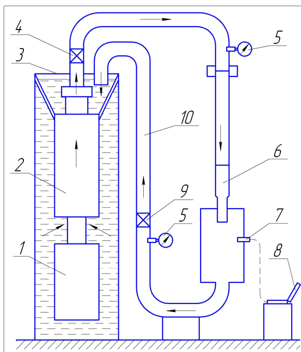
1 – електродвигун; 2 – відцентровий насос; 3 – ємність з робочою рідиною; 4 – кран; 5 – манометр; 6 – удосконалений гідравлічний генератор імпульсно-хвильової дії; 7 – п'єзокерамічний акустичний датчик; 8 – комп'ютер; 9 – кран; 10 – гідравлічна лінія
