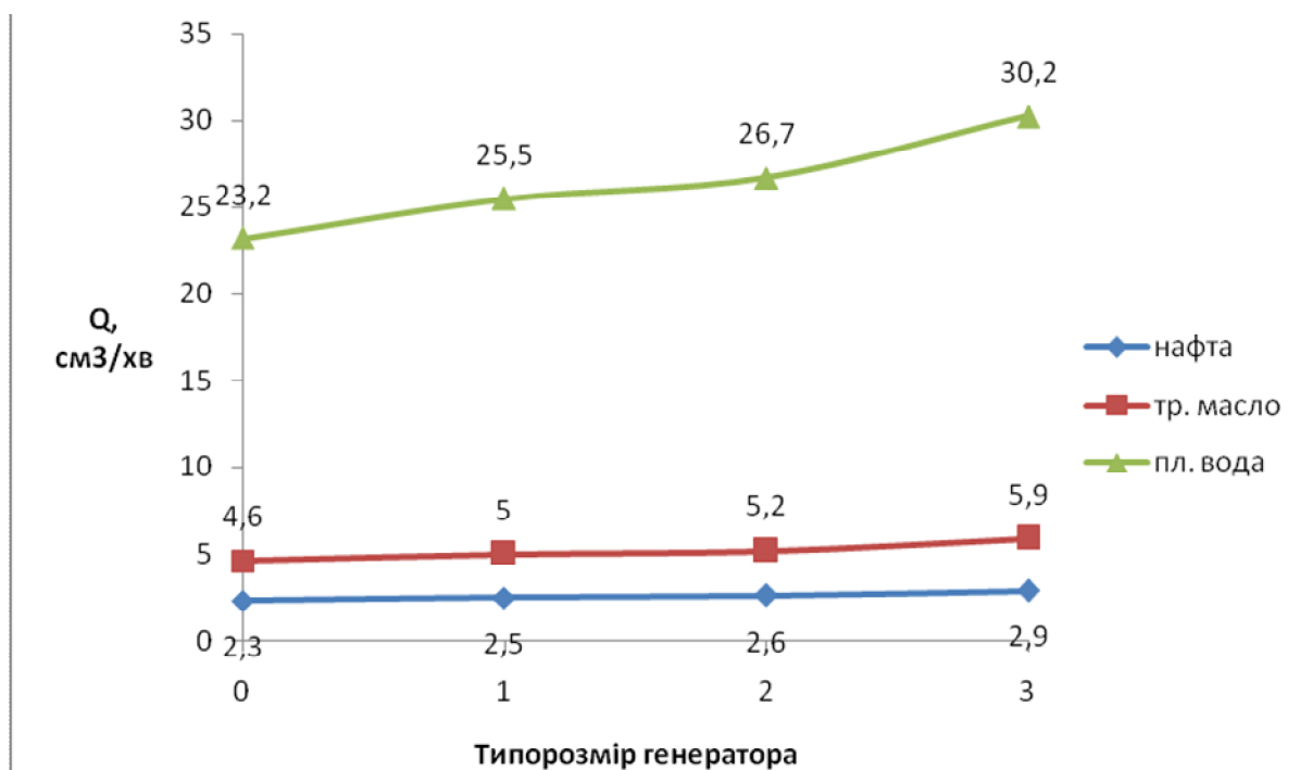
0 – фільтрація рідини без генератора, 1 – фільтрація рідини при роботі клапану довжиною 50%, 2 – фільтрація рідини при роботі клапану довжиною 70%, 3 – фільтрація рідини при роботі клапану довжиною 100%
