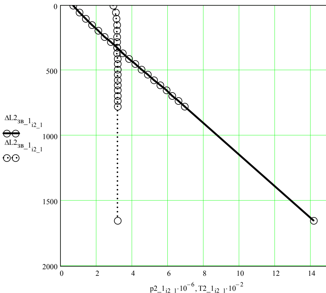
Рисунок 4 – Графіки розподілів тиску p і температури T газоводонафтового та водонафтового потоків вздовж колони насосно-компресорних труб відносно до глибини L_{Ні}
