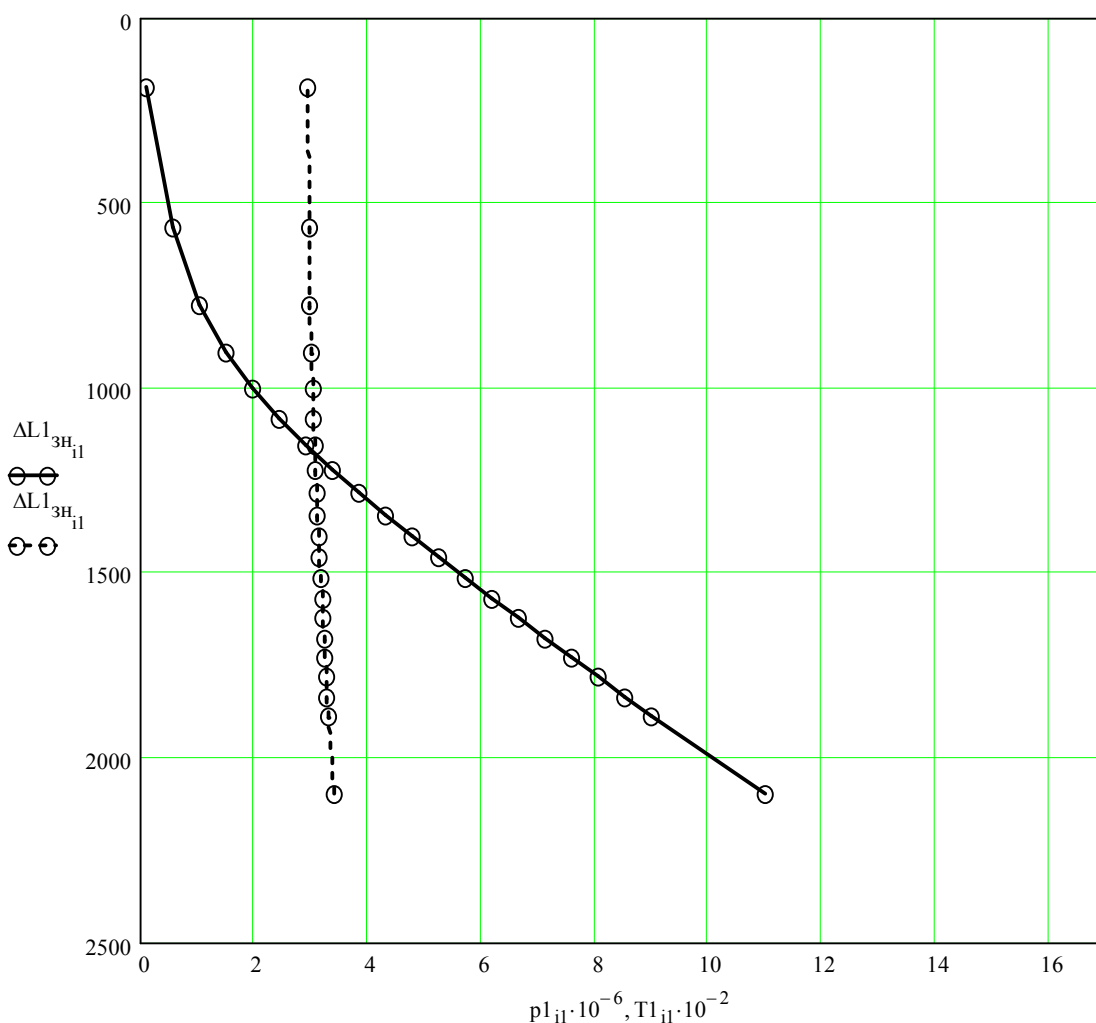
Рисунок 2 – Графіки розподілу тиску p і температури T водонафтового і газоводонафтового потоків вздовж експлуатаційної колони свердловини (за даними в розрахункових точках)
