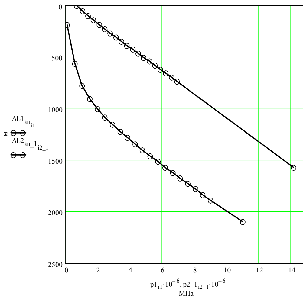
Рисунок 5 – Суміщені криві розподілів тисків p сумішей в експлуатаційній колоні та в НКТ
