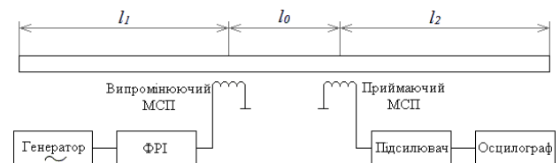
Рисунок 11 - Структура стенду для визначення основних характеристик і параметрів МСП та його елементів
