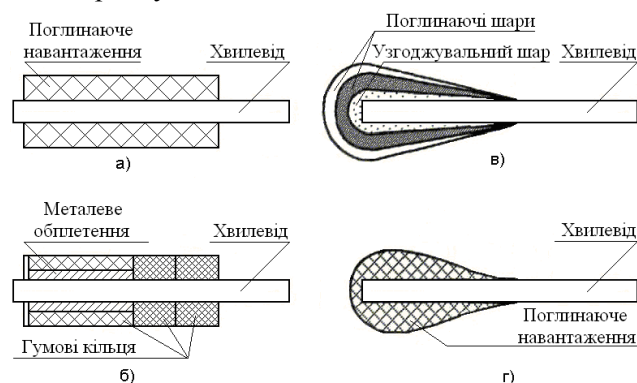
а)- циліндричний одношаровий, (б)-циліндричний багатоеlementний, (в) краплеподібний багатосаровий, (г) краплеподібний одношаровий
