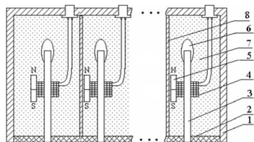
Рисунок 8 - Конструкція лінійки малоапертурних МСП
