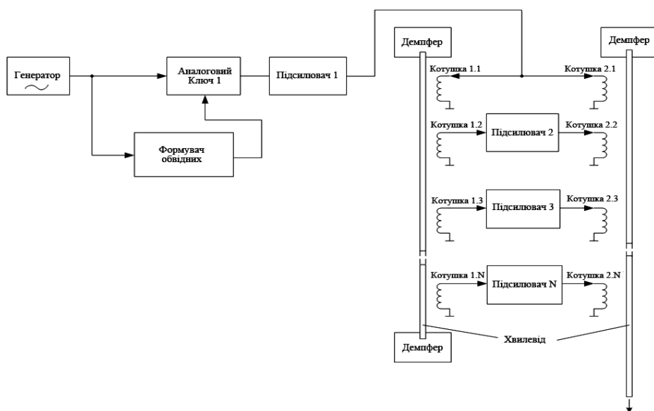
Рисунок 17 - Структурна схема блоку збудження широкопasmового МСП підвищеної потужності
