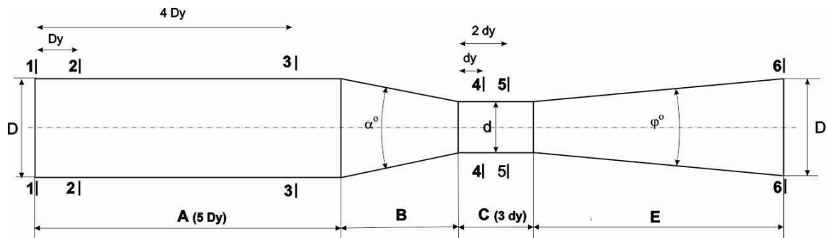
A - вхідна циліндрична ділянка, на якій встановлюється турбінний лічильник; B – конфузور; C - горловина, на якій встановлюється ультразвуковий лічильник; E – дифузор.
