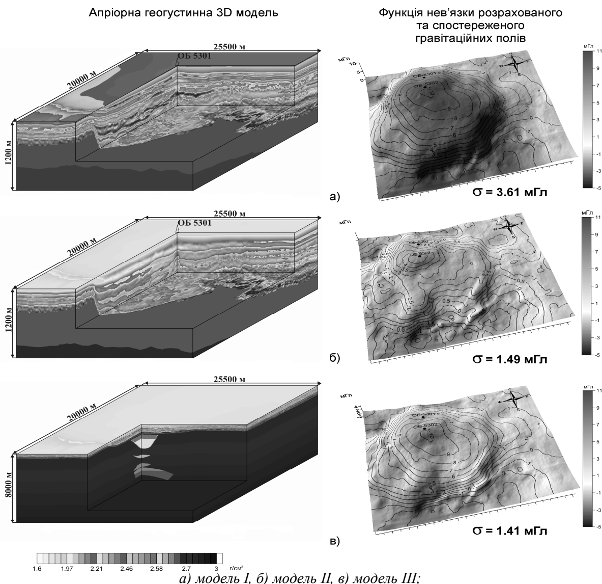
Рисунок 6 – Апріорні геогустинні моделі та розраховані гравітаційні поля
