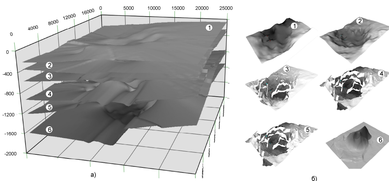
а) об'ємна модель, б) структурні карти по основних структурно-літологічних комплексах: 1 – J_{3ox} ; 2 – J_{2bt} ; 3 – J_{2bs} ; 4 – C_2b ; 5 – C_2b+T+PC ; 6 – PR
