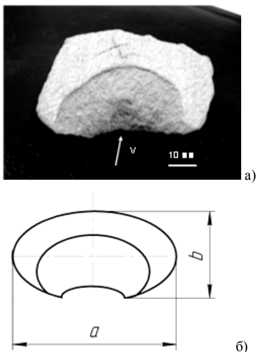
Рисунок 10 - Загальний вигляд фрагментів шламу, отриманих при різанні пісковіку Теревовлянського родовища різцем РП-221 при заданій глибині різання h_p = 8 мм і кроці різання H = 60 мм (а); V-вектор напрямку відколу частинки шламу і узагальнена схема фрагмента шламу (б)
