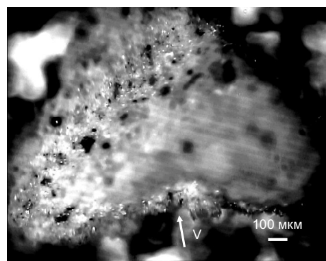
Рисунок 13 - Фрагмент шламу, отриманий в результаті різання блоку Торезького пісковіку алмазними зернами, закріпленими у вставці із Славутича (V-вектор напрямку відколу частинки шламу)
