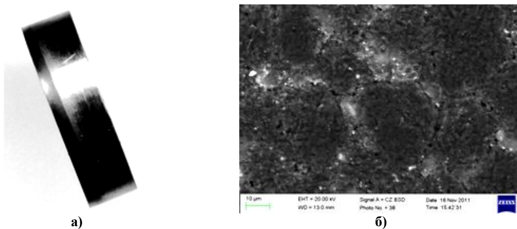
а – загальний вигляд; б – структура поверхні різальної кромки АТП
