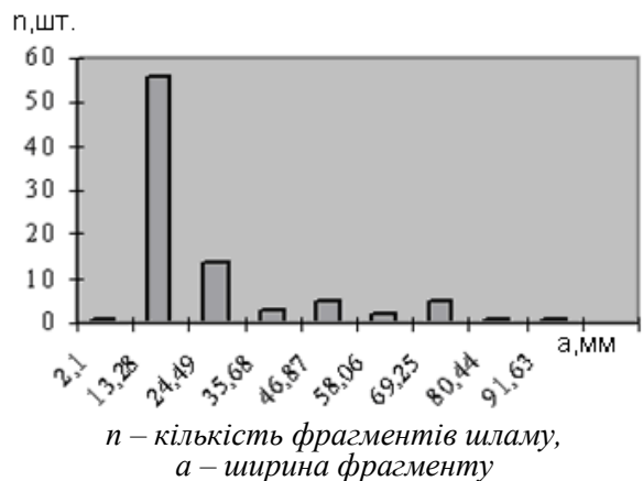
Рисунок 6 – Розподіл значень ширини фрагментів шламу, що утворюється в результаті різання різцем РП-221, оснащеним твердосплавною вставкою блоку пісковиків Теребовлянського родовища на глибину h р =8 мм з кроком різання H=60 мм
