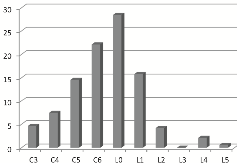
Рисунок 5 – Розподіл мол. % псевдокомпонентів для конденсату С (ТС [12], табл. II)
