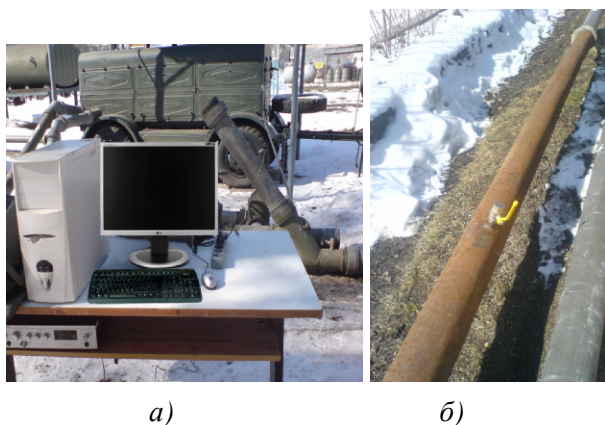
а) – система генерування та реєстрації сигналів, б) – модуль імітації витоку
