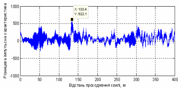
Рисунок 5 – Різницева характеристика трубопроводу, одержана для випадку наявності в трубопроводі витoku \varnothing 3 мм
