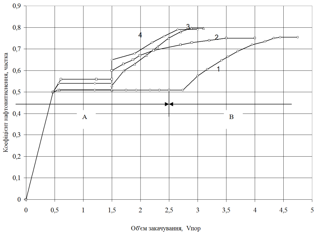
1 - зниження тиску при закритому виході з моделі пласта, витримування впродовж 24 год для розгазування та подальше нагнітання води (ділянка А); подальше зниження тиску при відкритому виході з моделі пласта та подальше нагнітання води (ділянка Б); 2 - одночасне нагнітання води та зниження тиску; 3 - зниження тиску з подальшим нагнітанням води (для умов менілітових відкладів Північно-Долинського родовища); 4 - зниження тиску з подальшим нагнітанням води
