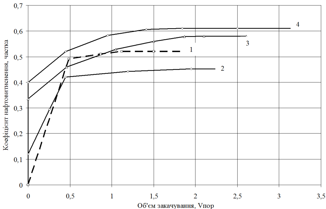
1 – крива витиснення нафти за пластового тиску ( R_{пл} ), вищого тиску насичення нафти газом ( R_{нас} ); 2 - крива витиснення нафти за пластового тиску R_{пл}=0,75 R_{нас} ; 3 – крива витиснення нафти при R_{пл}=0,5 R_{нас} ; 4 - крива витиснення нафти при R_{пл}=0,25 R_{нас}
