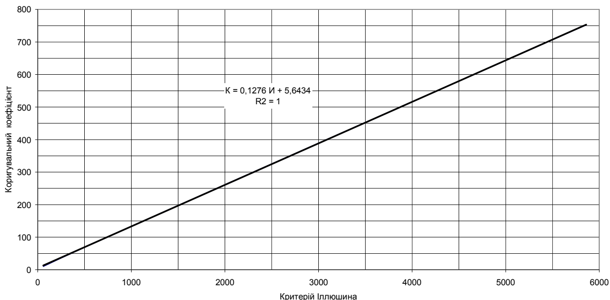
Рисунок 1 — Залежність коригувального коефіцієнта збільшення гідравлічного опору від критерію Іллюшина за ламінарного режиму ( Re=583 , пластична в'язкість нафти 0,04 Па·с)
