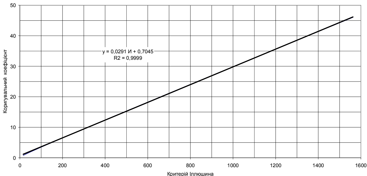
Рисунок 2 — Залежність коригувального коефіцієнта збільшення гідравлічного опору від критерію Іллюшина за турбулентного режиму ( Re=8738 , пластична в'язкість нафти 0,02 Па·с)
