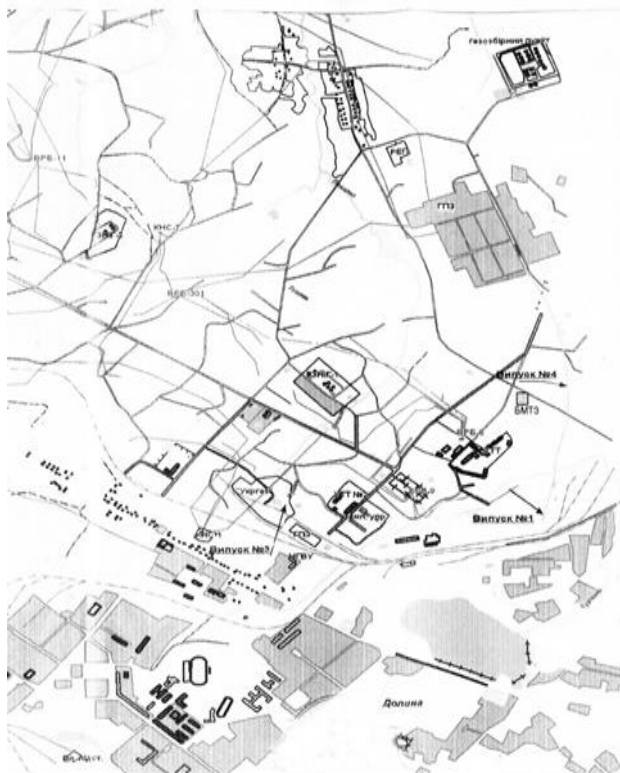
Рис. 1. Схема водовідведення стічних вод у річки Тур'янка та Луцава
