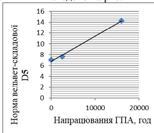
Рисунок 1 – Лінійна апроксимація залежності норми вейвлет-складової деталізації p'ятого порядку від часу напрацювання ГПА
