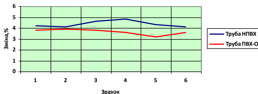
Рис.3. Графік зміни довжини труб з НПВХ і труб з ПВХ-О (150°C на протязі 20 хв)
