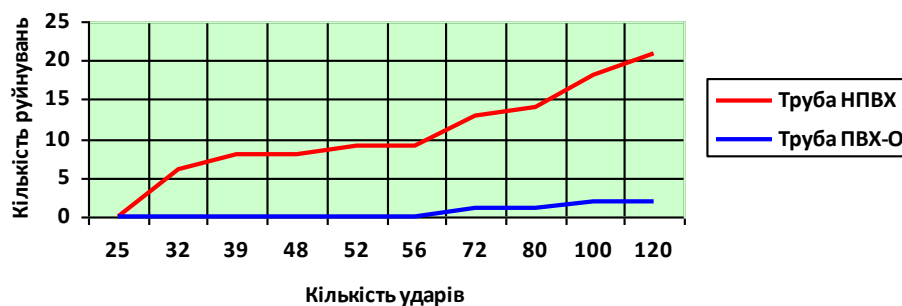
Рис.1. Графік руйнувань труб з НПВХ і труб з ПВХ-О в аналізі на опір удару падаючого вантажу
