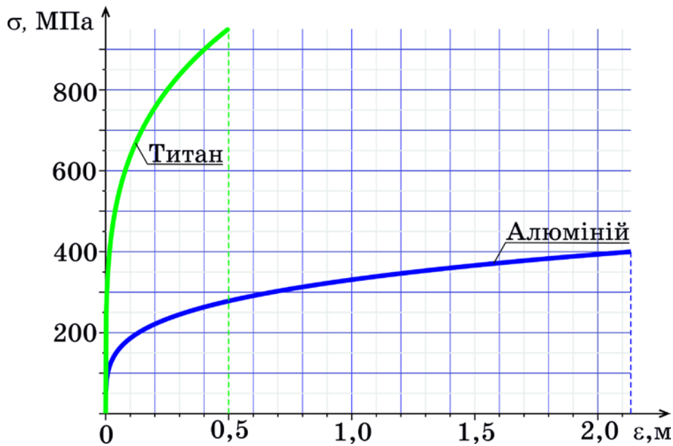
Рисунок 6.5 – Діаграма «напруження — деформація» бурових труб, виготовлених з титанових та алюмінієвих сплавів
