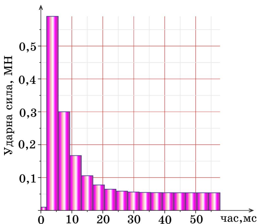
Рисунок 6.2 – Ударний імпульс в зоні прихоплення
