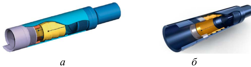
Рисунок 1.14 – Овершот, що застосовують для вилучення [73; 159]
