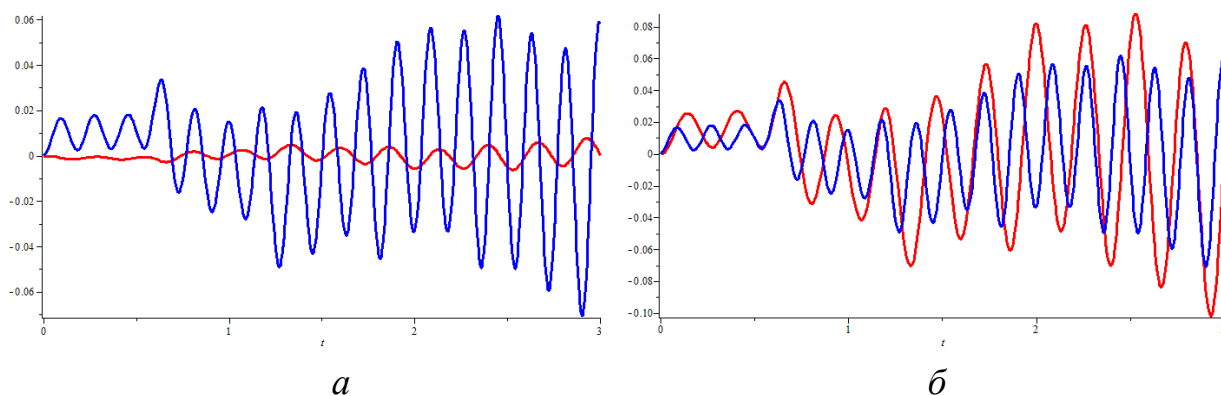
Рисунок Г.15 – Поздовжні коливання аварійної компоновки БК у місці встановлення осцилятора: a – вільні, б – вимушені при налаштуванні на третю (червона крива) і четверту (синя крива) власну частоту
