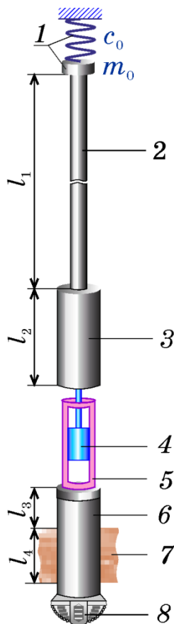
Рисунок 4.1 – Розрахункова схема бурильної колони з вмонтованим ударним механізмом
